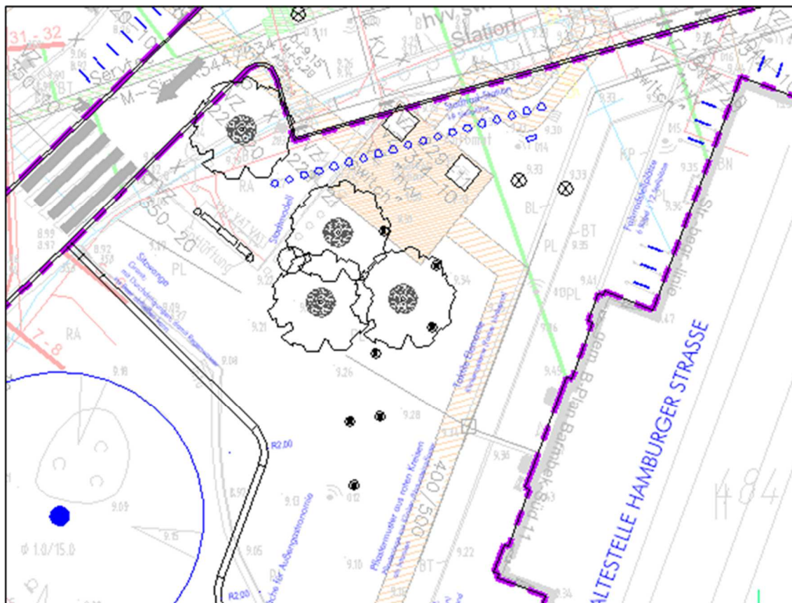
Abbildung 13: Lageplanausschnitt mit Darstellung der unterirdischen Fernwärmanlagen und Elektroleitungen
