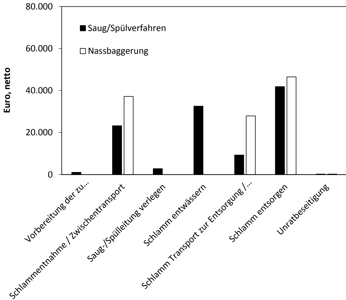
Abbildung 2: Kostenschätzung Nassbaggerung und Saug-/Spülverfahren nach Einzelpositionen im Gliederungspunkt „Schlammmentnahme, Transport, Entsorgung“ des LV
