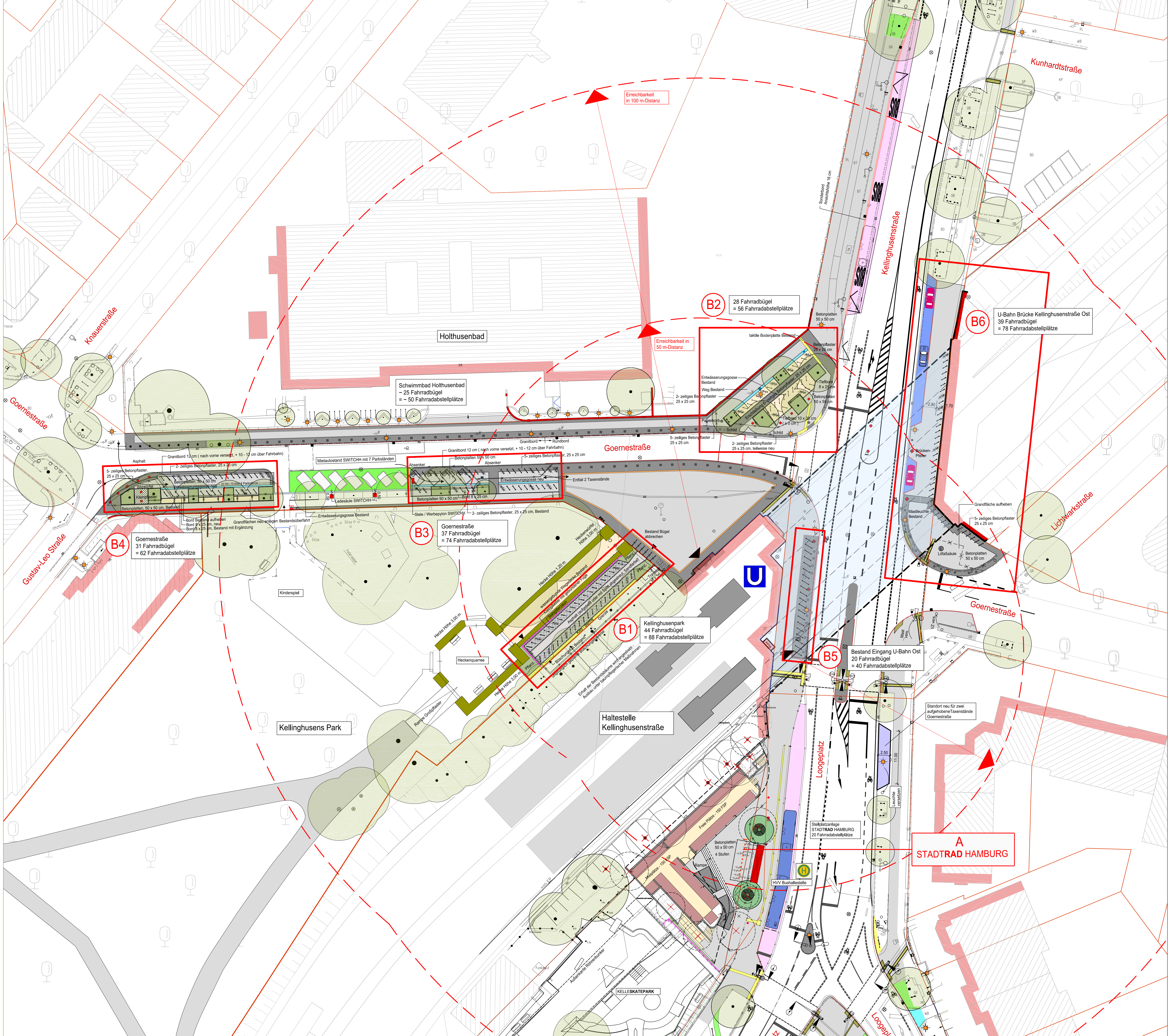
Plandarstellung Plattenflächen
