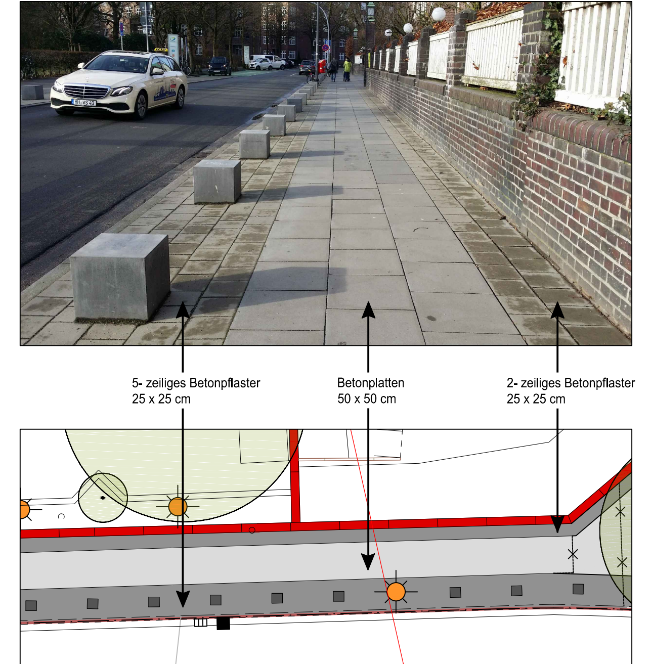
Plandarstellung Plattenflächen
