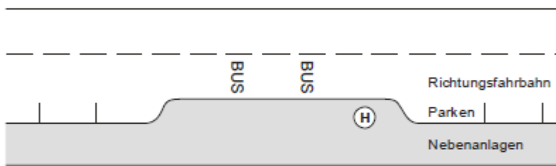
Abb. 3: Prinzipskizze Buskap, ZVBN 2014.
