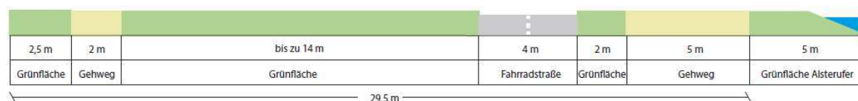
Abbildung 5: Aufteilung und Abmessung des zukünftigen Straßenquerschnitts vor Hausnummer 30 (Planung)
