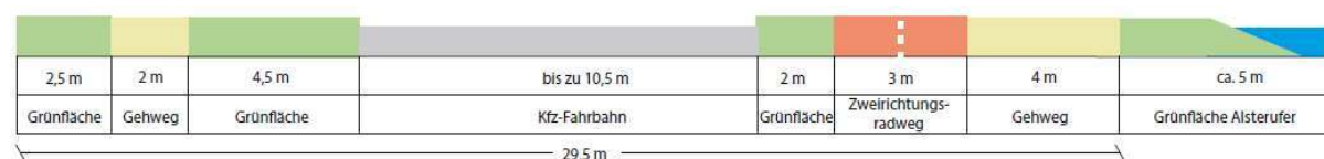
Abbildung 3: Aufteilung und Abmessung des Straßenquerschnitts vor Hausnummer 30 (Bestand)
