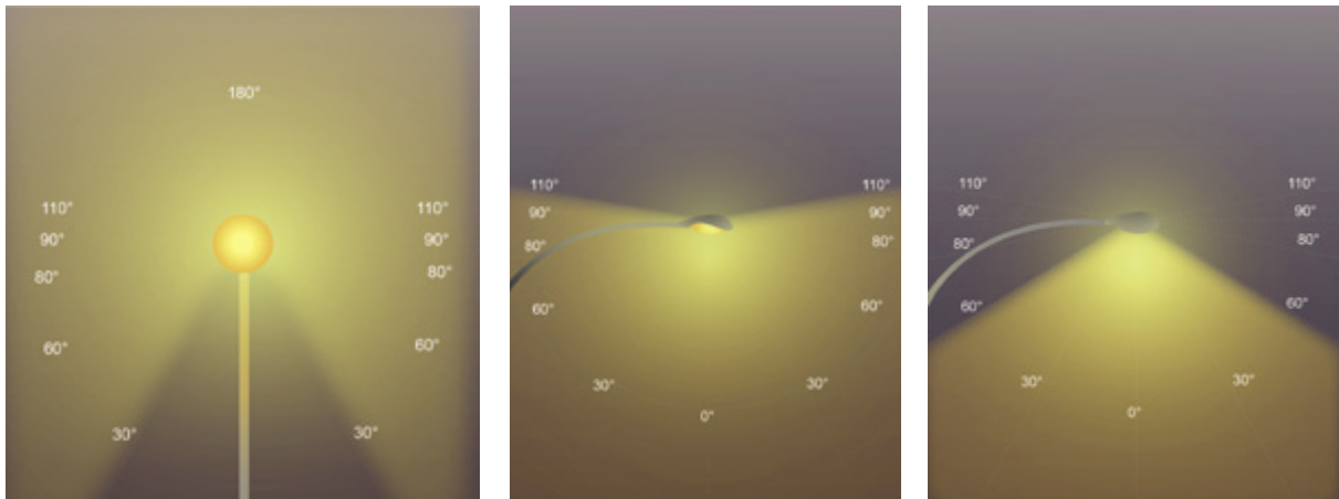
Abb. 13: Abstrahlungswinkel unterschiedlicher Leuchten. Die Gradzahlen beziehen sich auf den Winkel zur Vertikalen. Das rechte Bild zeigt die naturschutzfachlich beste Option mit einem engen Lichtkegel, der weniger als 60^\circ zur Vertikalen aufweist. Illustration von Catherine Perez Vega aus Schroer et al. (2019).
