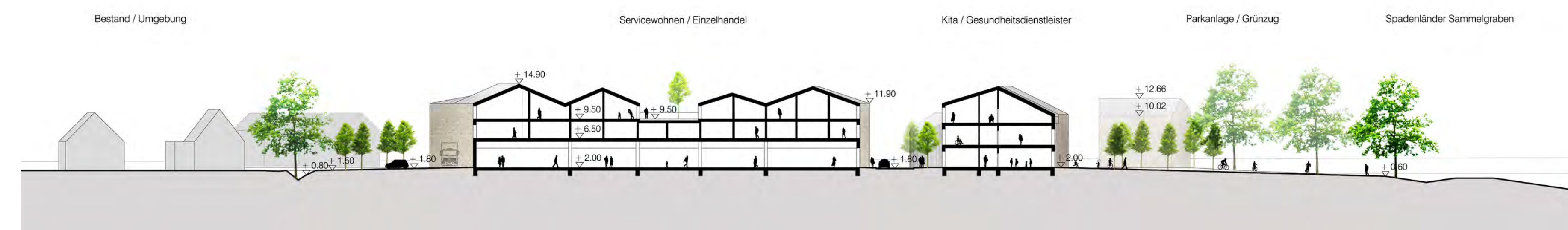
SCHNITT 4-4
