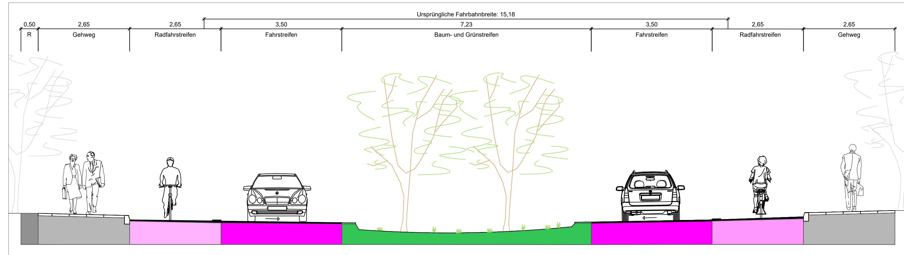
Querschnitt 3
