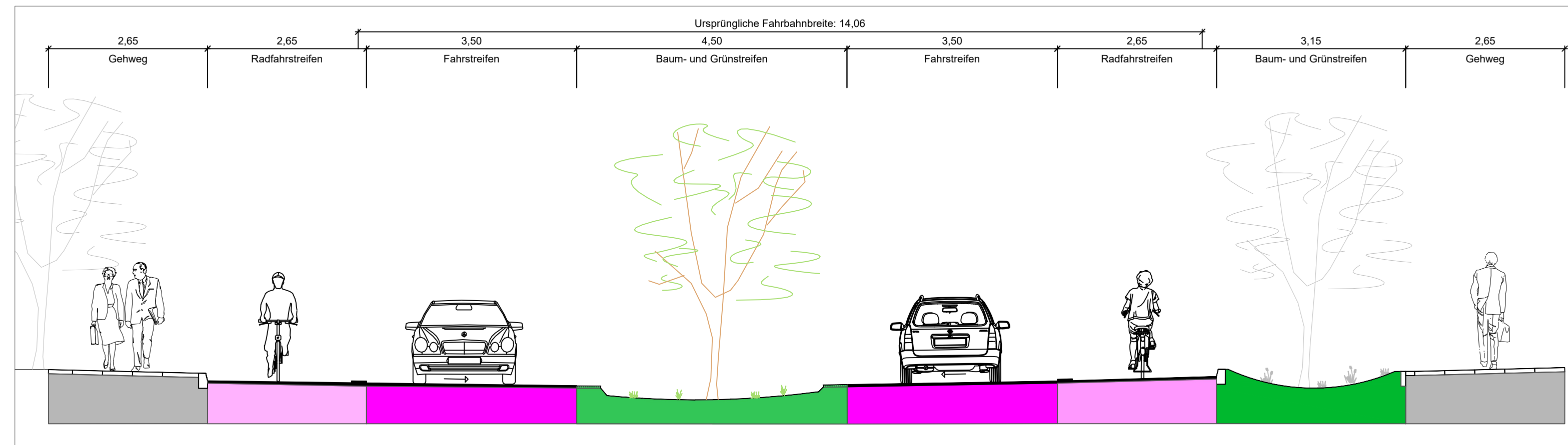
Querschnitt 2
