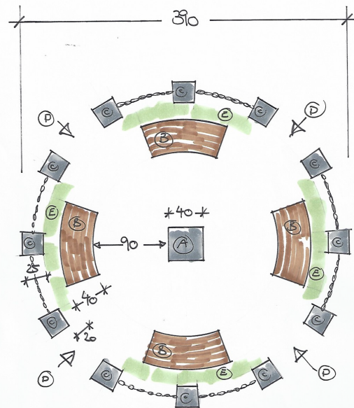
DRAUFSICHT ANLAGE
