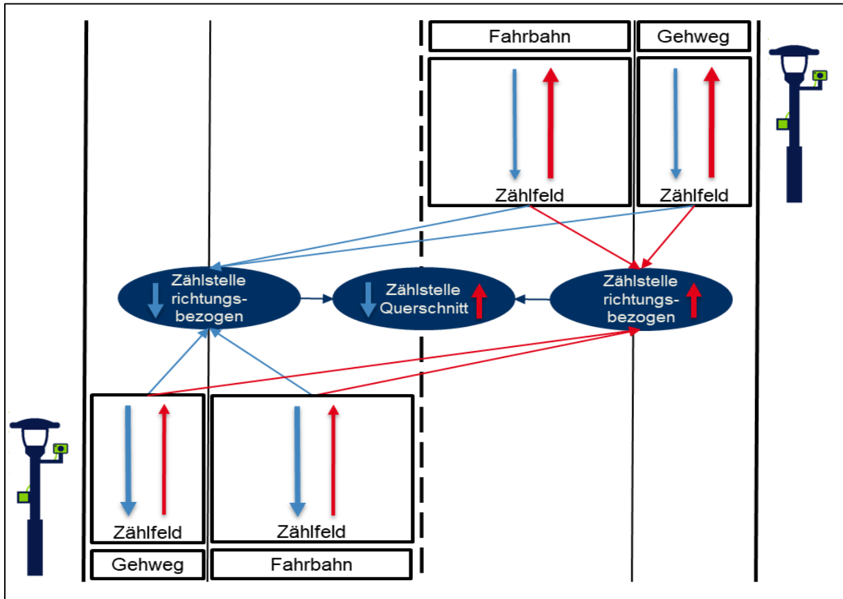
Abbildung 1: Schematische Darstellung des Zählstellenaufbaus
