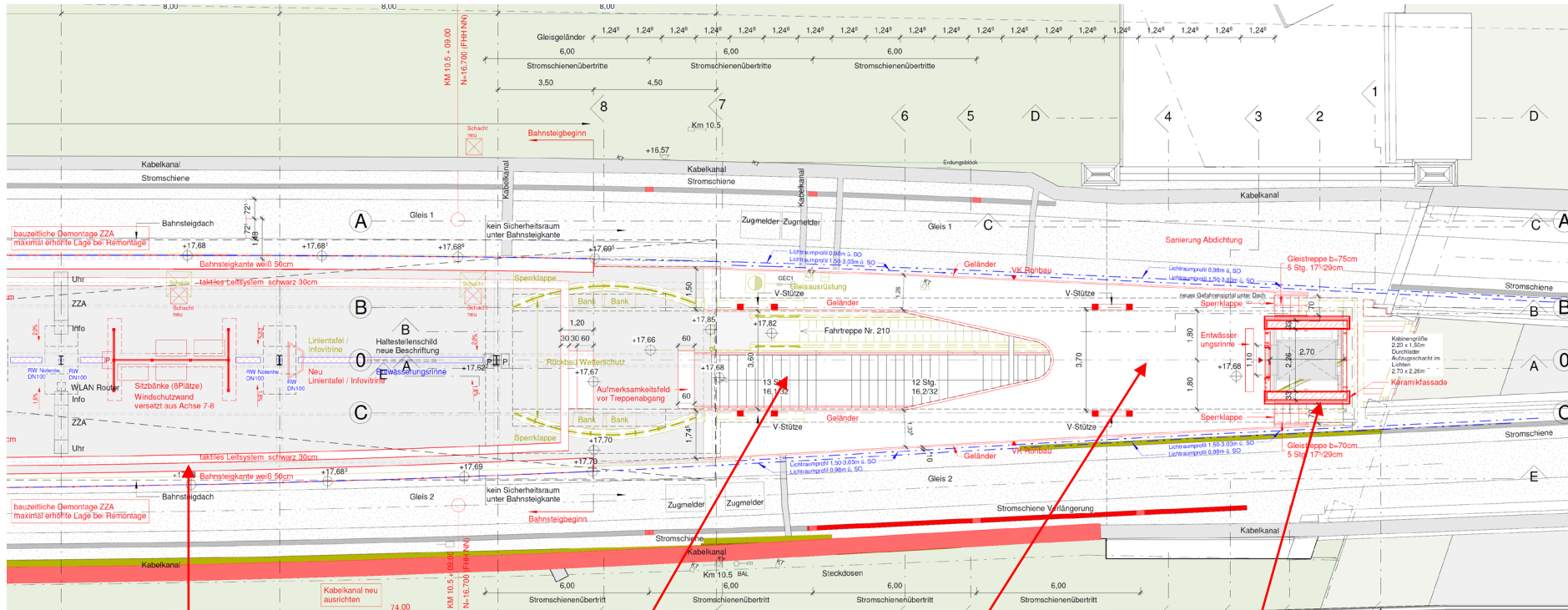
Grundriss Bahnsteig
