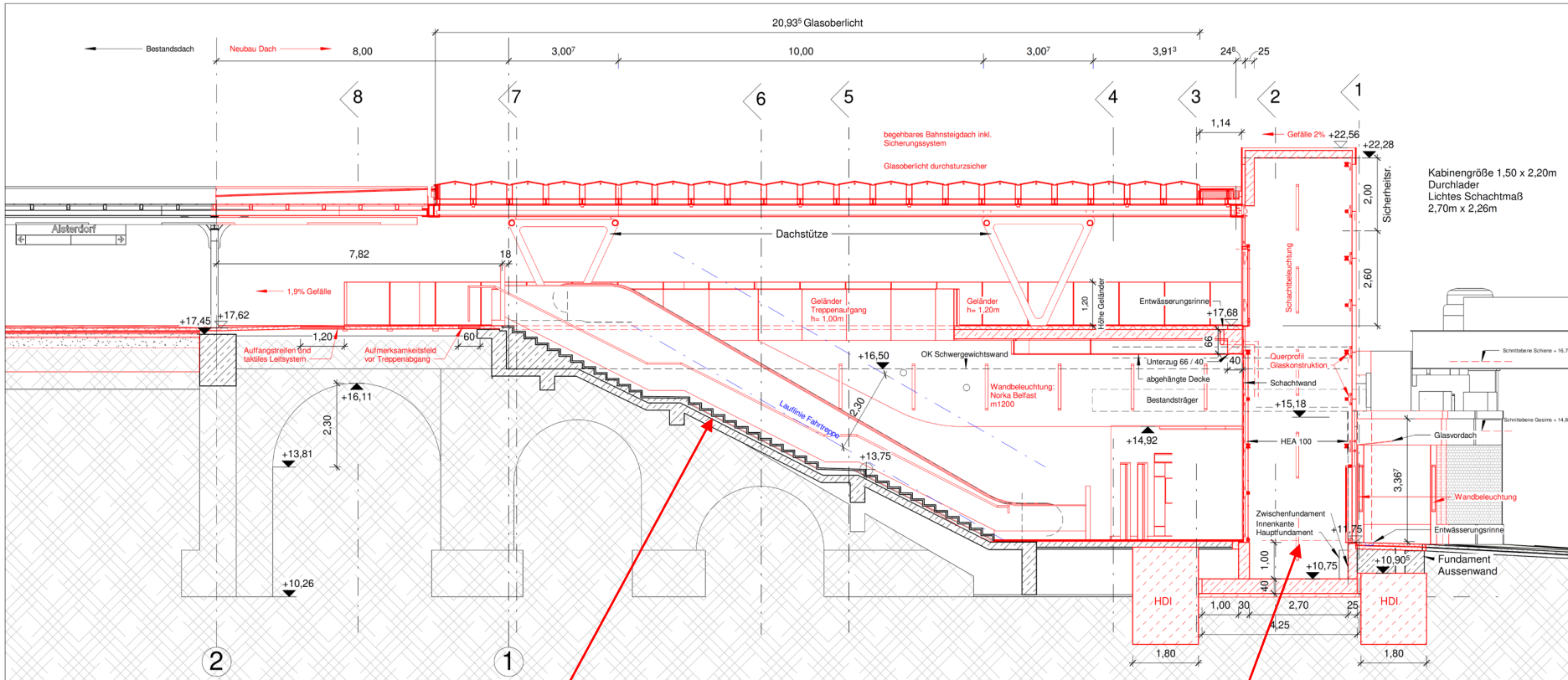
Schnitt A-A
